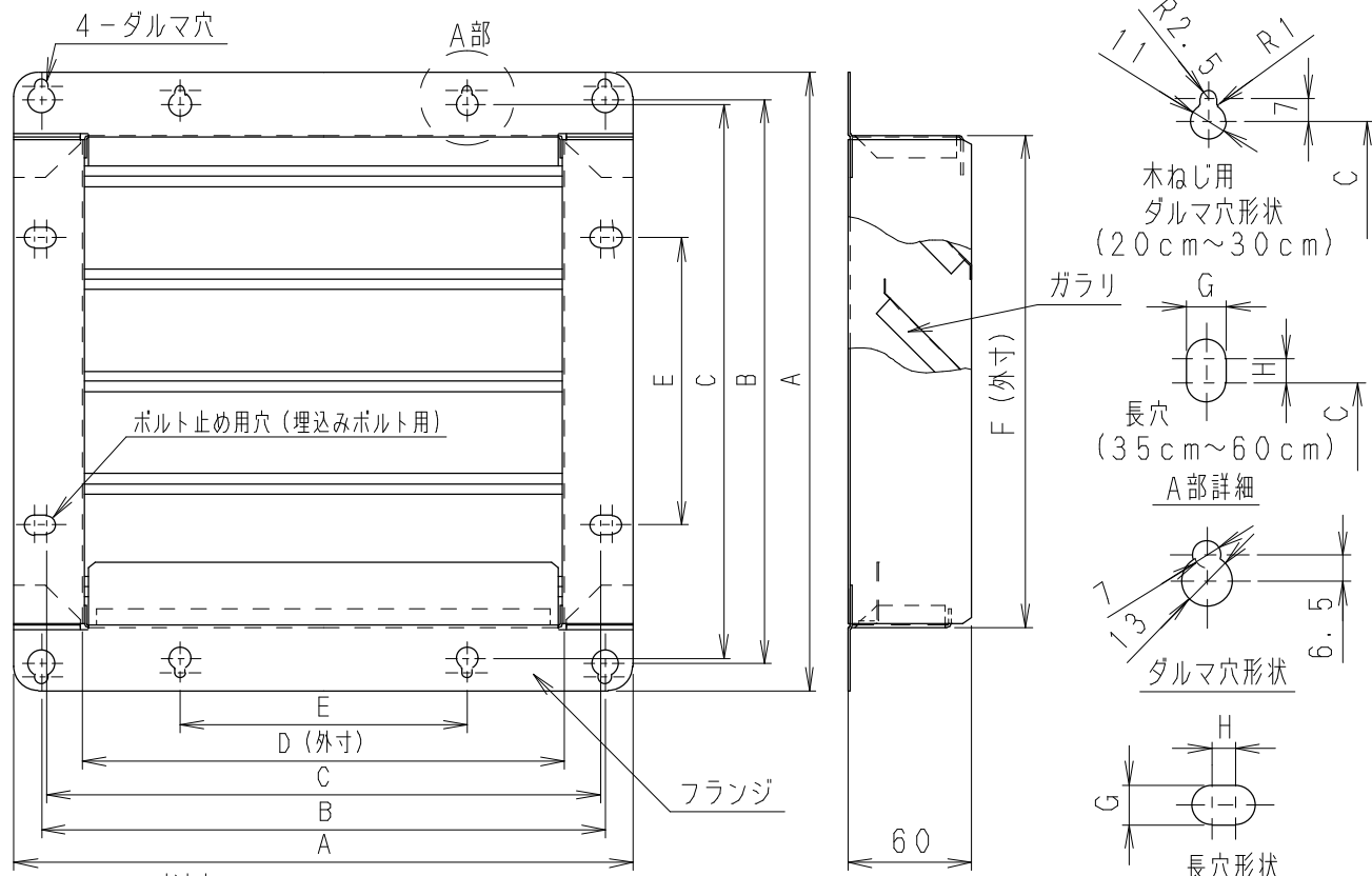
■ 寸法表
