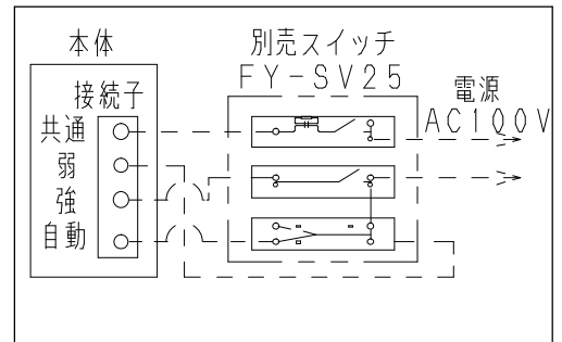
■結線図
