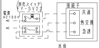
■結線図
