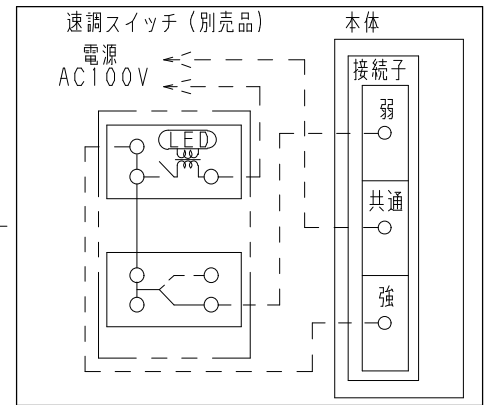
■結線図
