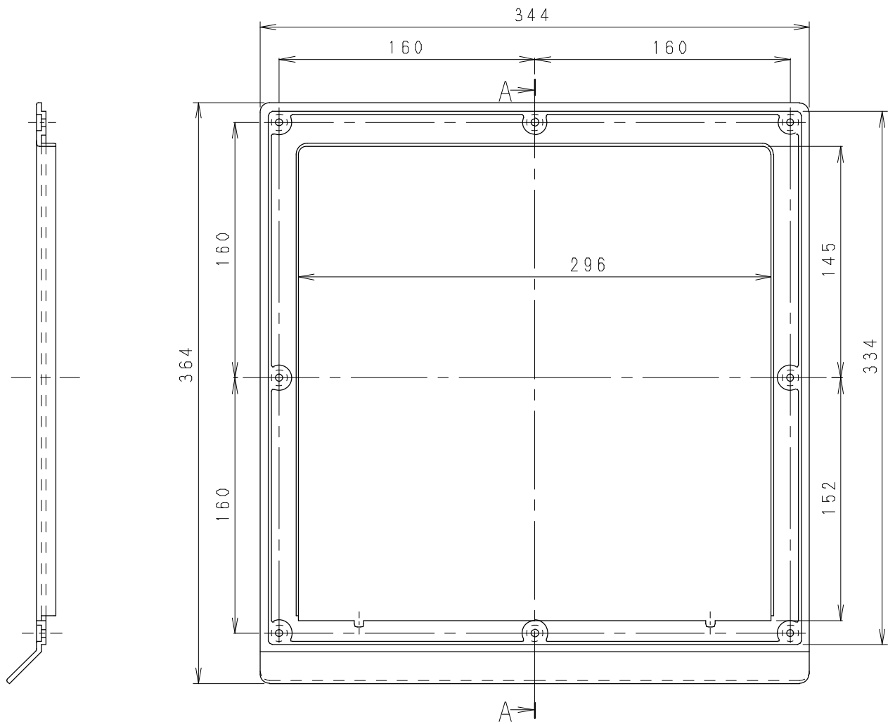
A-A SEC.
