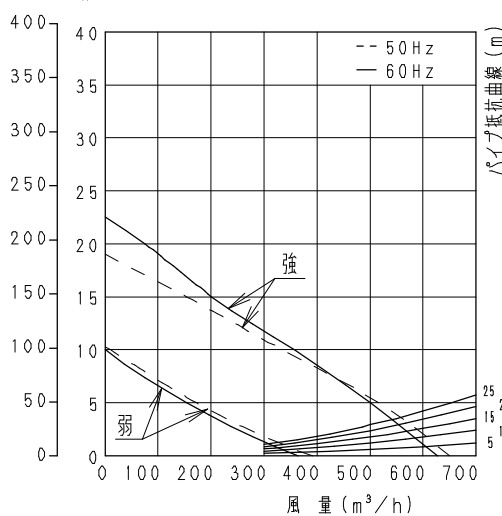
■ 静圧-風量特性曲線
